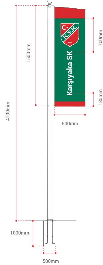
Mafsallı Döner Tip Gönder Bayrak
